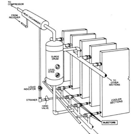
Multi. Chiller Sections (crit. charge)
